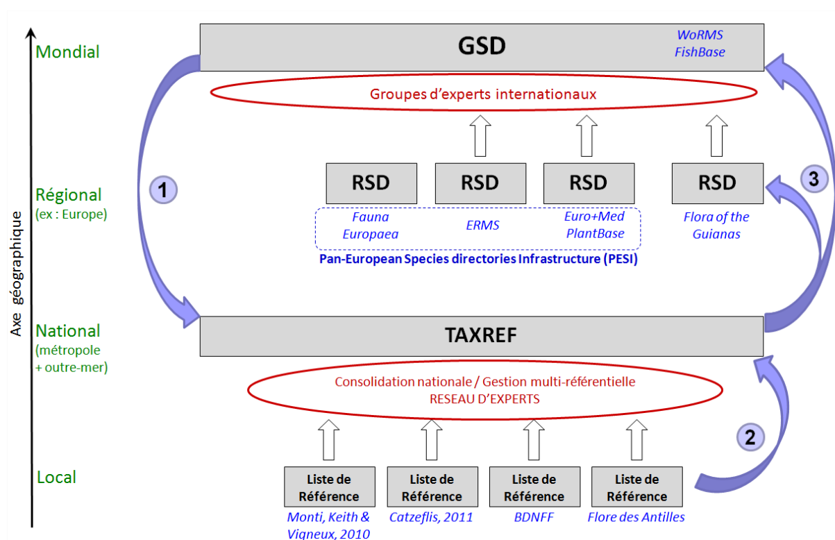
Figure 3: Interaction entre TAXREF et les référentiels existants.
