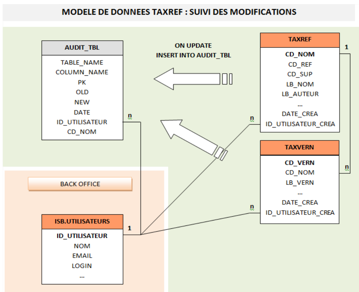
Figure 9 : Modèle de données de TAXREF : schéma du suivi des modifications.
